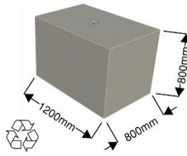
C3Cblock™ 1288SL Slät översida
