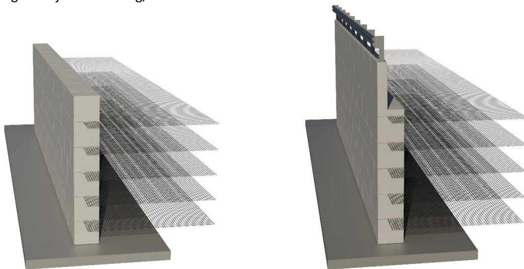
Figur 5.2g-h. Stabilisering med geonät genom jordförankring.
