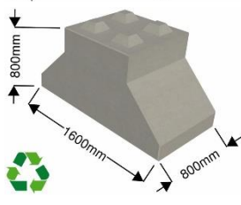
C3Cblock™ 1688DSF-1_R Dubbelsidigt Fundamentsblock Utbrett marktryck RETURBETONG
