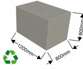
C3Cblock™ 1288SL_R Slät översida RETURBETONG
