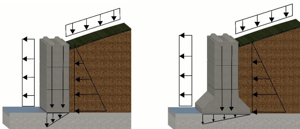
Figur 6.5a-b. Triangulärt marktryck.
